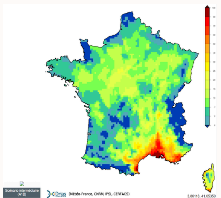
Nombre de jours de feux de forêts en 2040
