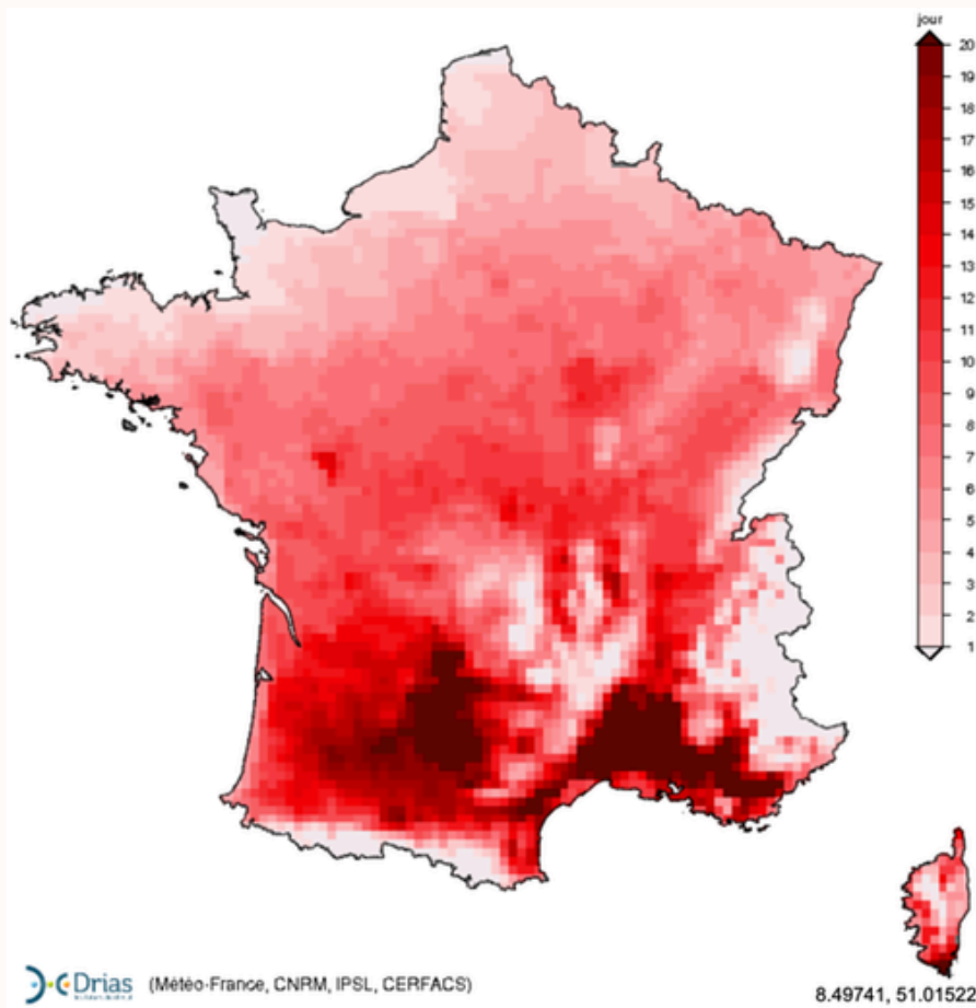
Nombre de jours de canicules en 2040
