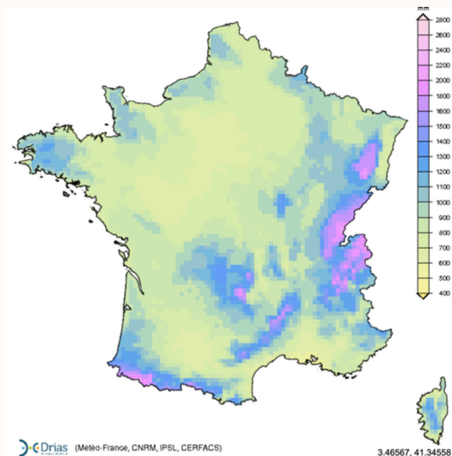
Cumul des précipitations annuelles en 2040
